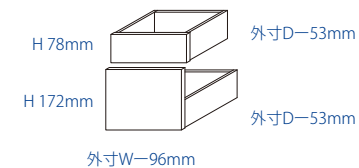
〈内引出付深型引出 H320〉
